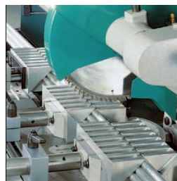
Tillbehör: Löstagbara backar på skruvstycket
